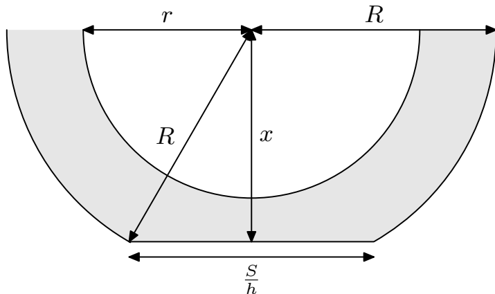
Obr. 1: Náčrtek k výpočtu vzdálenosti x země od středu kola.
